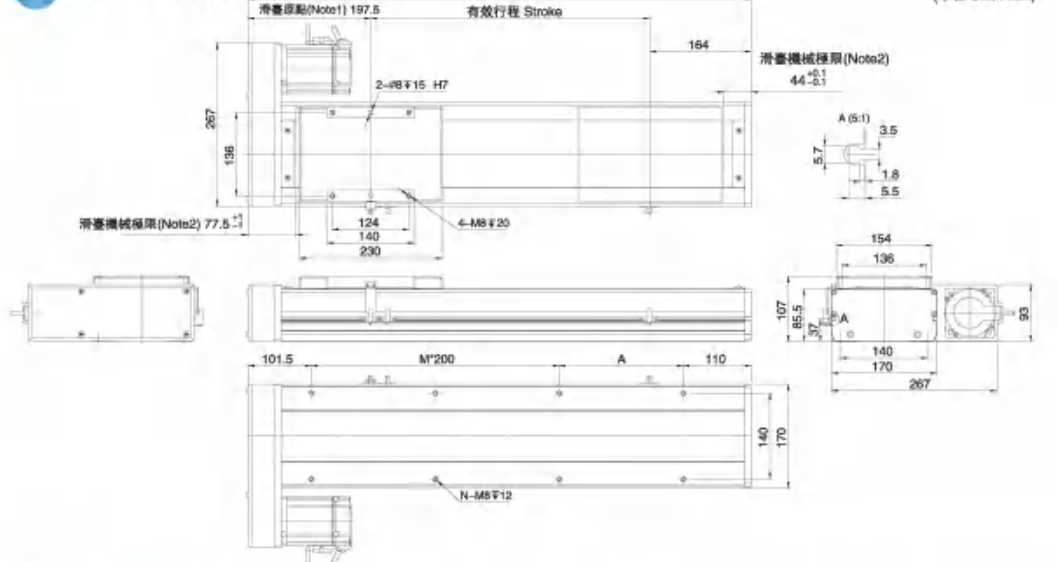
BR 馬達右折 Motor Right Side
