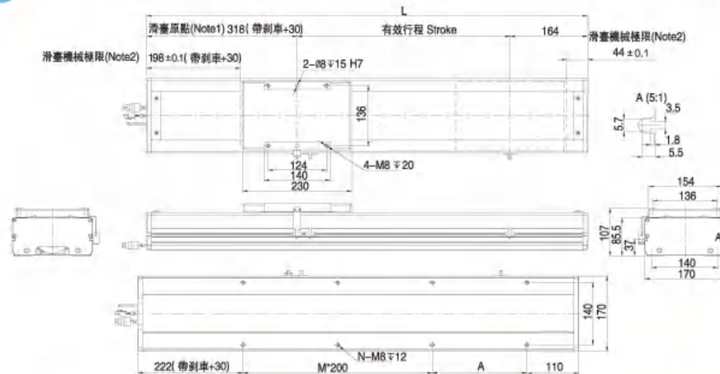
M 馬達直結 Motor Built-in
