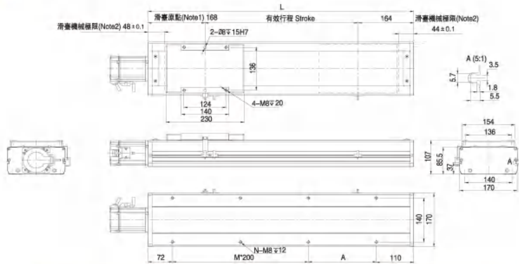
BC 馬達外露 Motor Exposed
