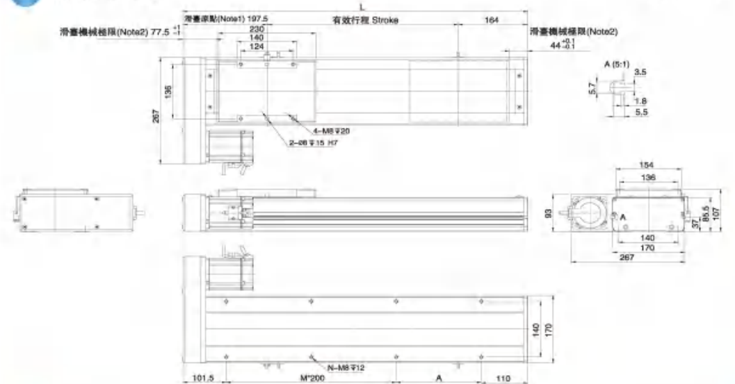
BL 馬達左折 Motor Left Side
